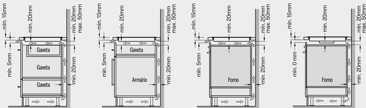
Distâncias mínimas para a ventilação correta
